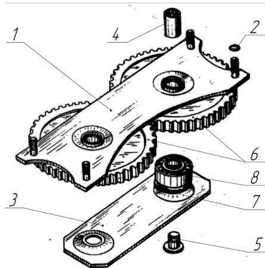
Рис. 2Г КДН 04.030 Блок шестерен
