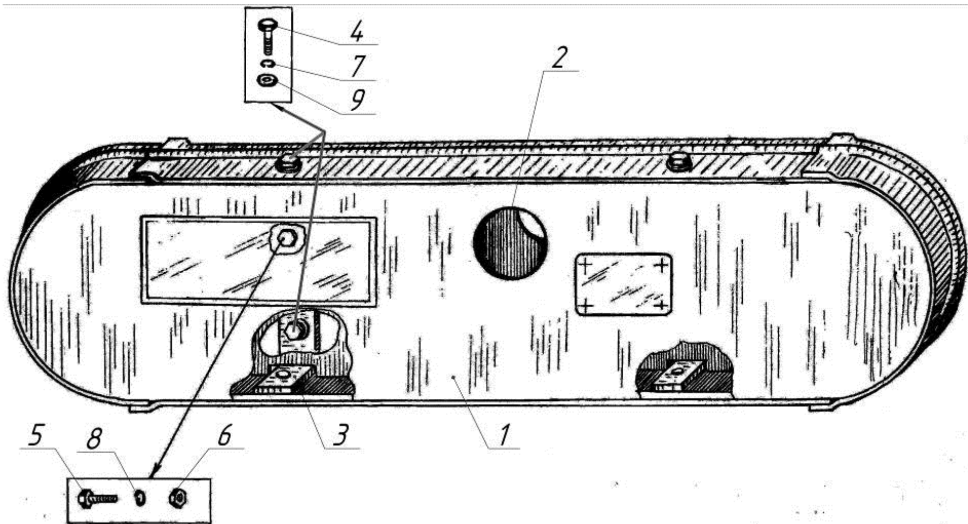
Рис. 7 КДН 01.000 Кожух
