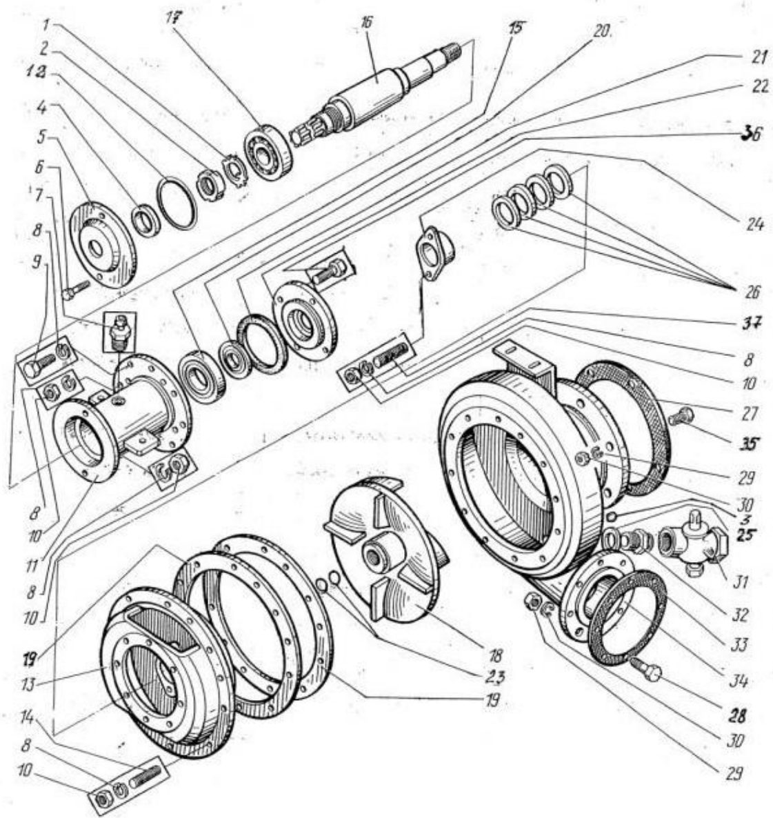
Рис. 13 – Насос (МЖТ16.40.00.000-01)
