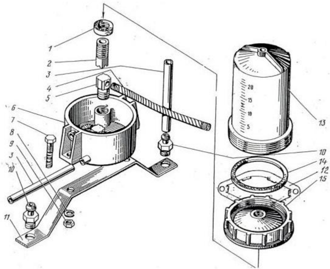
Рис 16 – Масленка (УВА 12.100)
