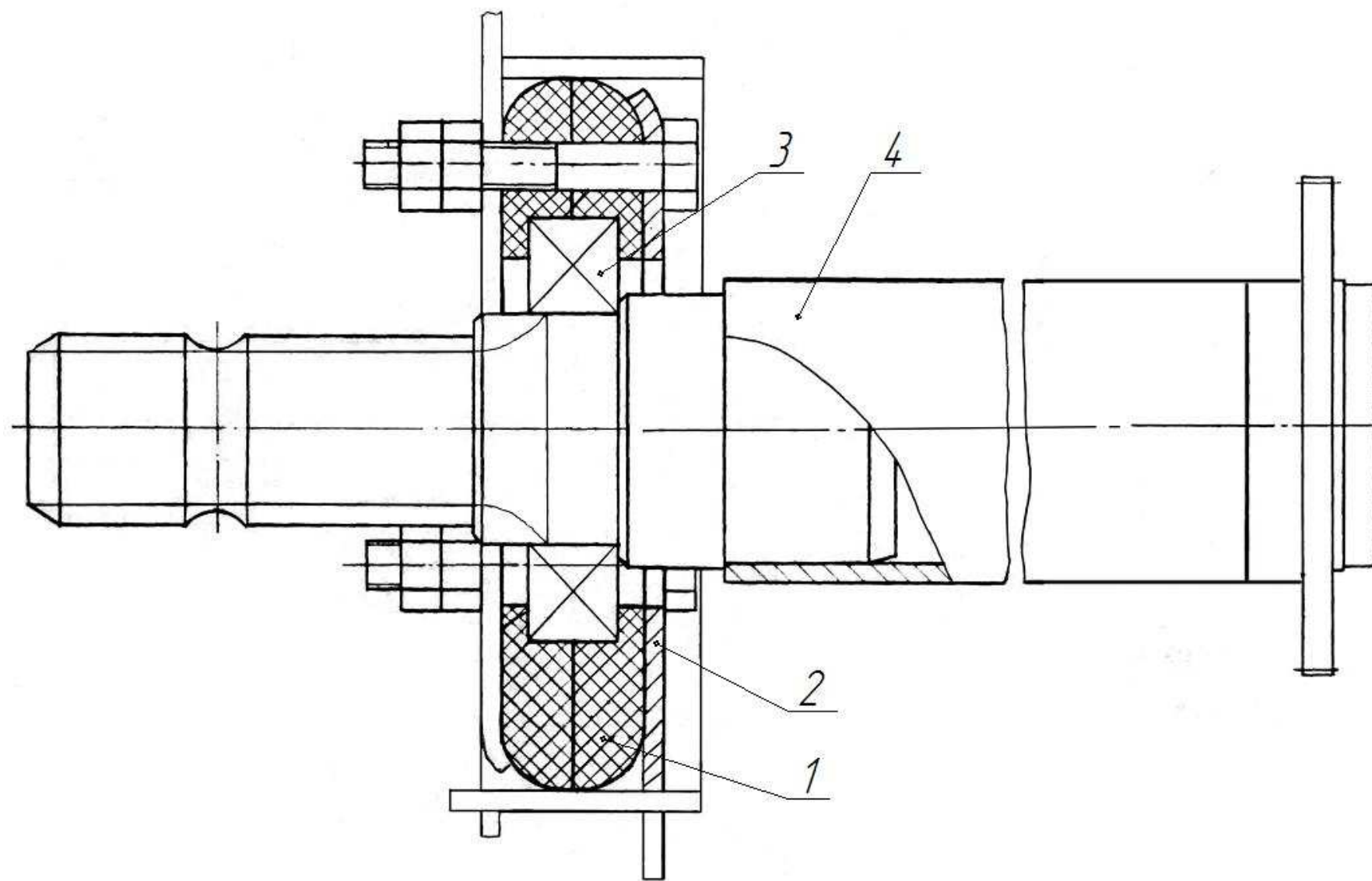
Рисунок 6 Вал передний
