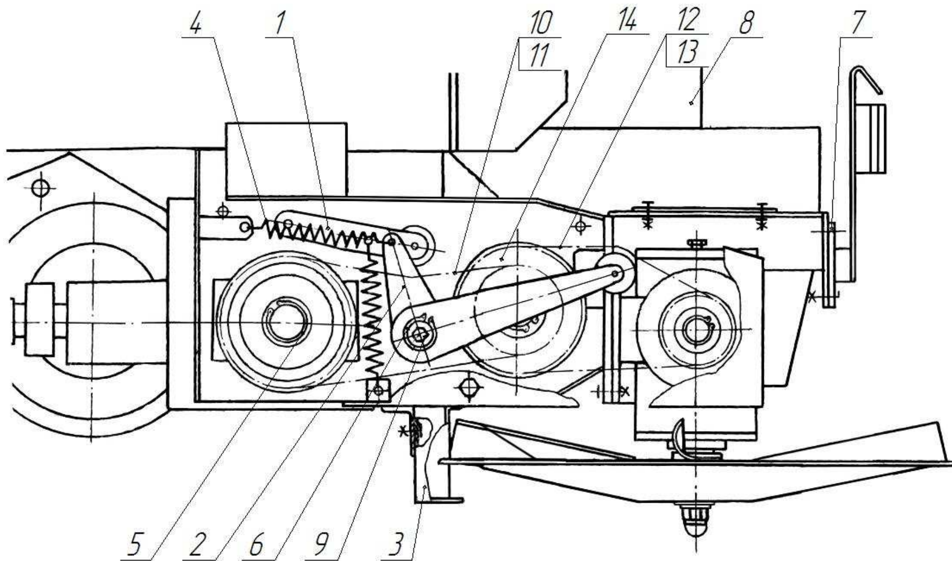
Рисунок 14 Передача цепная
